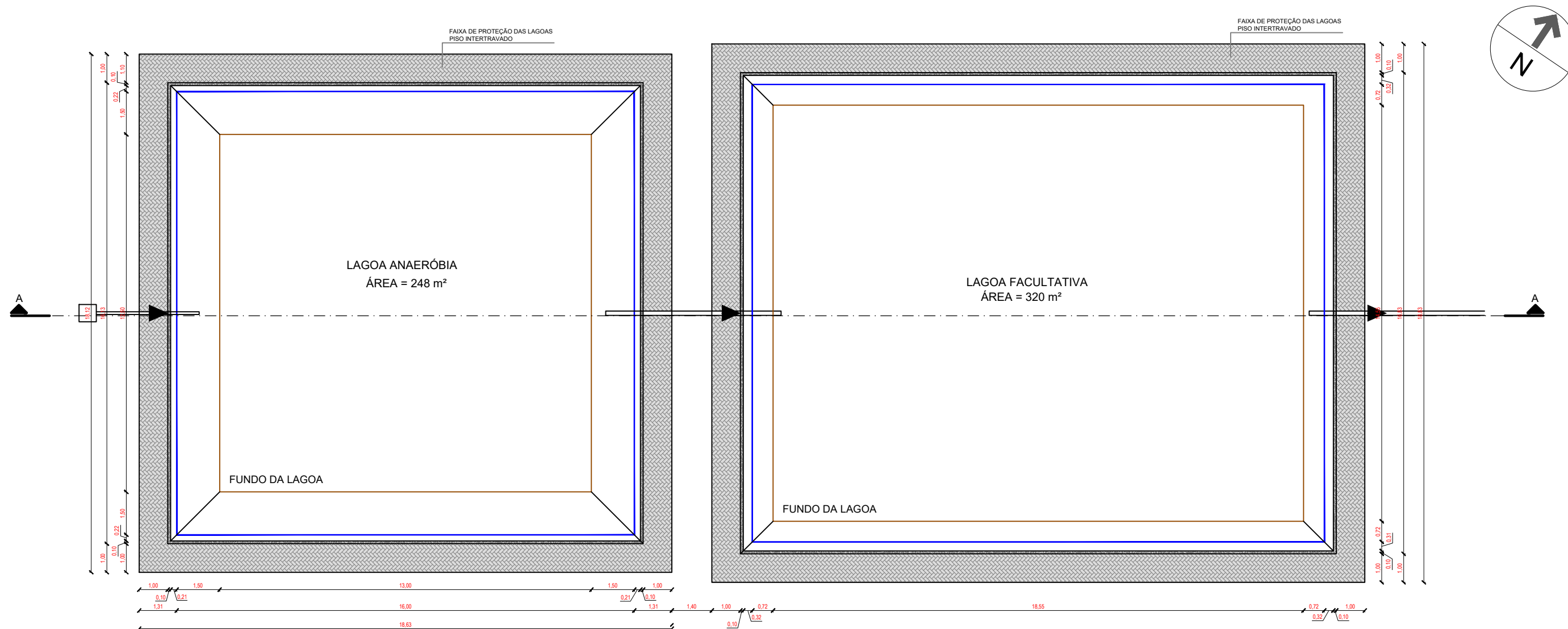
PLANTA BAIXA _ LAGOAS ESCALA _____ 1/150
